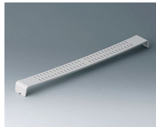
A0126370 Вставка, с вентиляционными отверстиями АБС (UL 94 HB) белый RAL 9002
