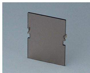
B6601580 Лицевая панель, 2 модуля, исп. VI ПК (UL 94 V-0) тонируемый 32x42mm
